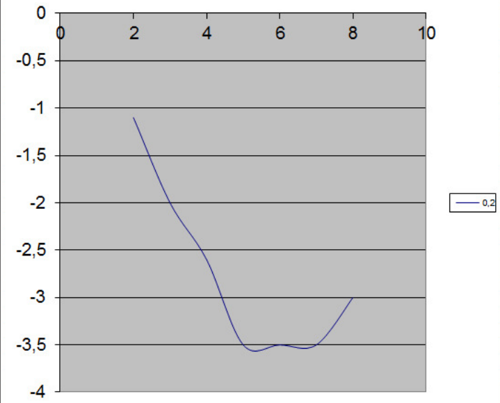
Lenkradmoment vs. Querbeschl.
